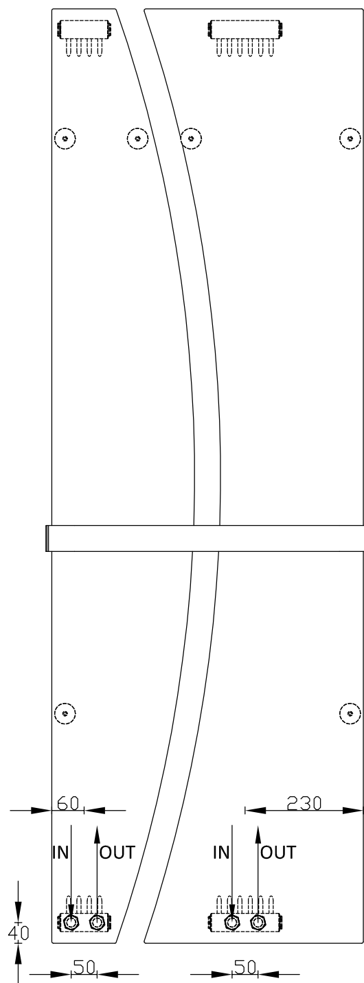
Vista frontale - Front view - Vue de face
